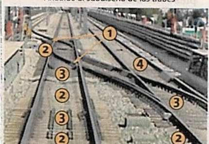
Posibles causas que colaboraron en falla de estructura Añadido al subdiseño de las traves
